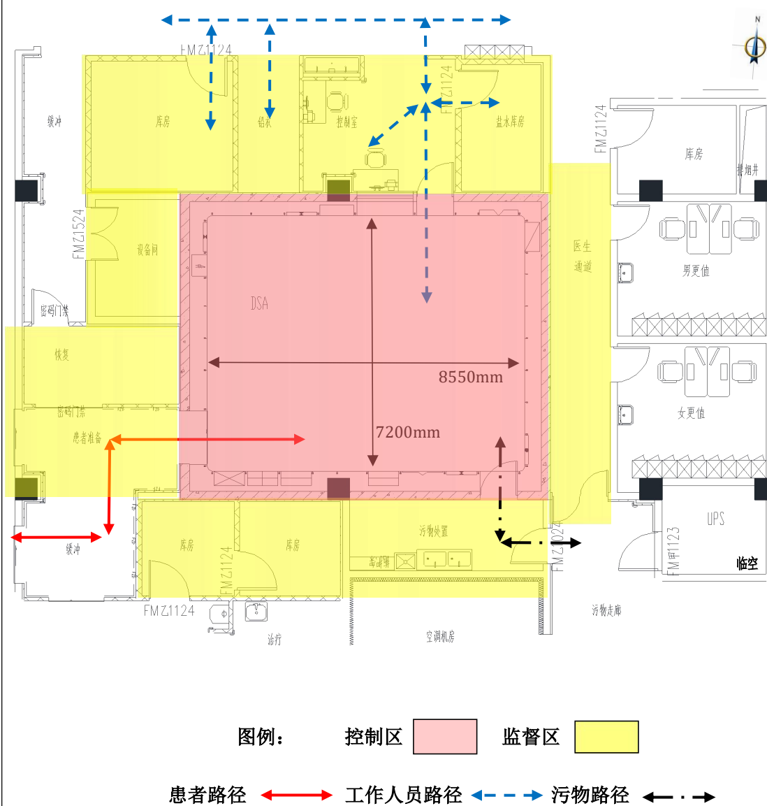
图 10-1 机房平面布局及辐射场所分区示意图
