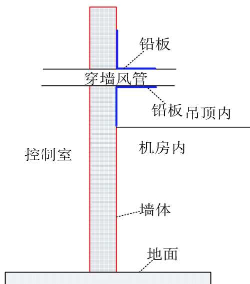
图10-2 风管穿越屏蔽墙体示意图
