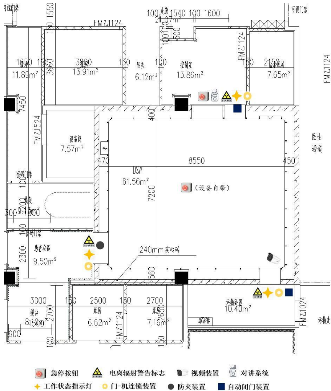
图 10-4 辐射防护设施分布图
