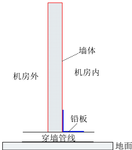
图 10-1 线缆穿墙示意图
