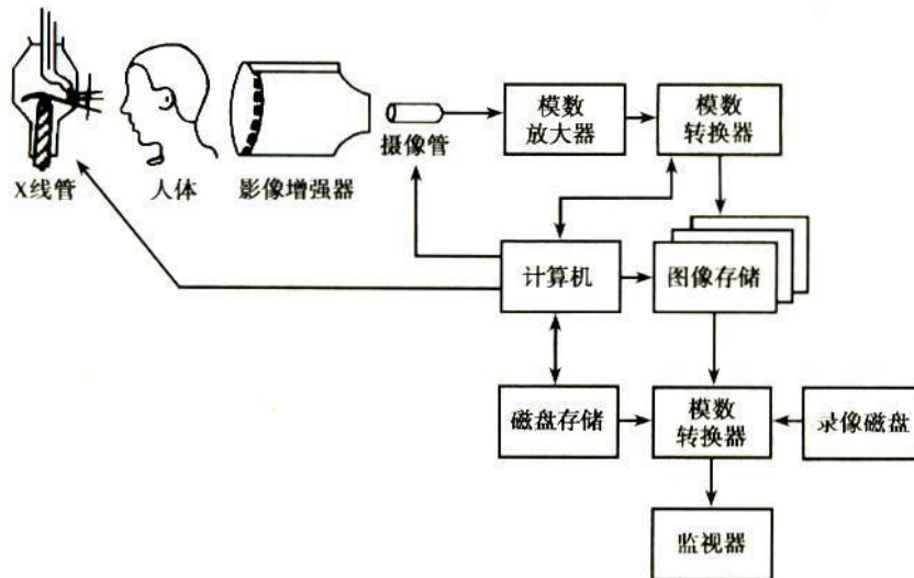
图 9-2 DSA 系统结构示意图
