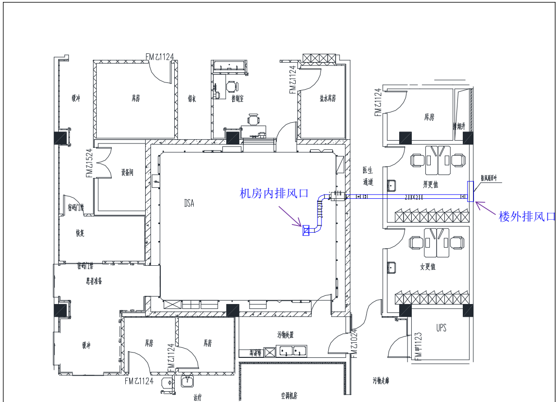
图 10-3 排风口及排风管道示意图
